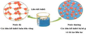
Hình 2: Mật độ các phân tử nước ở trạng thái rắn và lỏng
