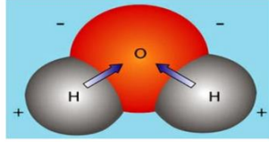
Hình 1 : Cấu trúc hoá học của nước
