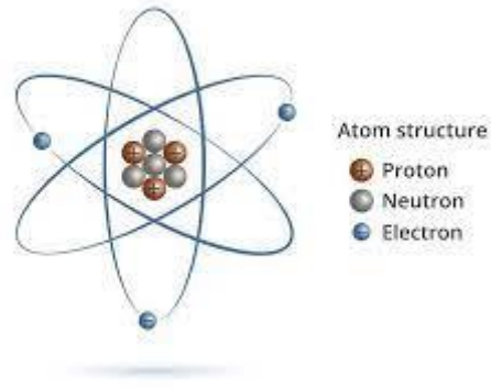
Hình cấu trúc Nguyên tử
