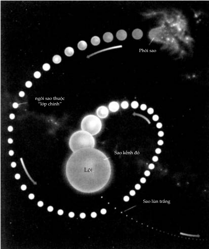
Hình 44. Sự ra đời, cuộc sống và cái chết của Mặt trời. Hình này cho thấy sự tiến hóa theo thời gian của Mặt trời (hướng thời gian được chỉ bằng mũi tên). Mặt trời sinh ra như một phôi sao, cách đây 4,55 tỉ năm, từ sự co mạnh lại của một đám mây khí giữa các vì sao. Ngay khi Mặt trời bắt đầu tổng hợp hiđrô thành hêli trong lõi của nó, nó trở thành một sao thuộc "lớp chính" và hiện nay nó vẫn như vậy. Pha này sẽ tiếp diễn trong phần lớn cuộc đời của Mặt trời. Trong khoảng 4,5 tỉ năm nữa, Mặt trời sẽ cạn kiệt nhiên liệu hiđrô trong lõi của mình và bắt đầu sử dụng nguồn dự trữ hiđrô trong lớp bao quanh lõi. Lớp vỏ bọc sẽ phồng lên khoảng một trăm lần kích thước hiện nay và Mặt trời sẽ trở thành một sao kình đỏ. Khi hiđrô bị cạn kiệt, nó sẽ bắt đầu sử dụng nguồn dự trữ nhiên liệu hêli. Giai đoạn sao kình đỏ sẽ rất ngắn. Sau khoảng 500 triệu năm, do cạn kiệt nhiên liệu nên sao kình đỏ sẽ suy sụp dưới tác dụng của lực hấp dẫn của chính nó để trở thành một sao lùn trắng có kích thước bằng Trái đất: đó chính là cái chết của Mặt trời. Sao lùn trắng sẽ tiếp tục bức xạ yếu ớt trong nhiều tỉ năm nữa. Bức xạ này không đến từ các phản ứng hạt nhân mà từ nhiệt bị cầm tù trong lõi nó trong khi xảy ra sự tổng hợp hạt nhân. Cuối cùng, khi nguồn dự trữ nhiệt cạn kiệt, sao lùn trắng sẽ trở thành một sao lùn đen không nhìn thấy được và sẽ gia nhập hàng ngũ vô số các xác sao nằm rải rác trong thiên hà.
