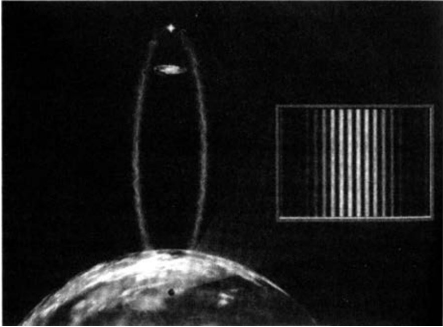
Hình 36. Một phiên bản vũ trụ của thí nghiệm khe Young. Ánh sáng của một quasar rất xa bị lực hấp dẫn của một thiên hà nằm giữa Trái đất và quasar làm lệch và chia thành hai chùm, và tụ tiêu lại trên Trái đất. Về nguyên tắc, các nhà thiên văn trên Trái đất có thể quan sát được các vân giao thoa.
