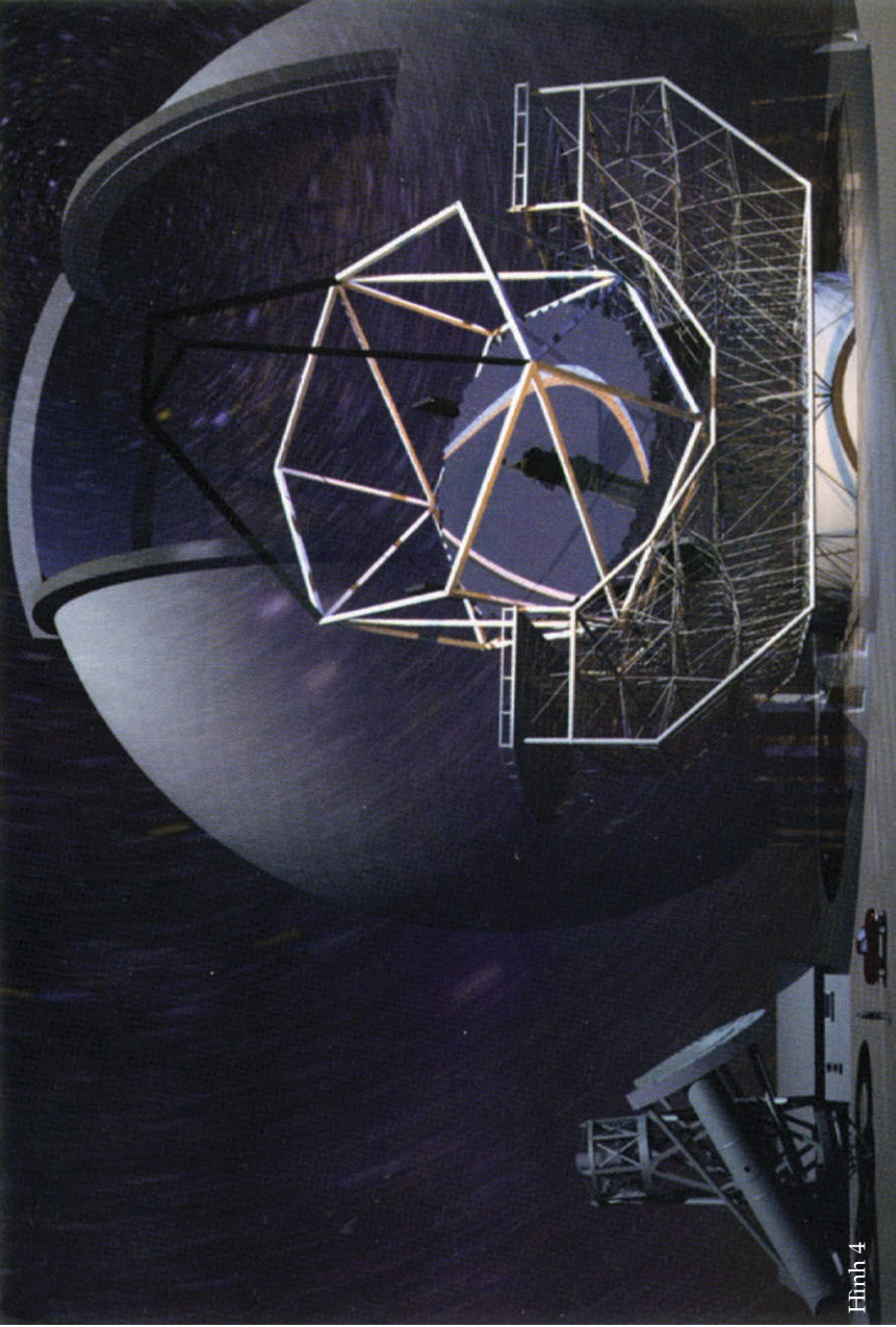
Các kính thiên văn khổng lồ của tương lai. Để lần ngược trở lại theo thời gian khoảng 13 tỷ năm và chiêm ngưỡng sự ra đời của những ngôi sao và thiên hà đầu tiên, các nhà thiên văn đã hăm hở bắt tay lập kế hoạch xây dựng những kính thiên văn khổng lồ trong tương lai. Một trong những dự án xây dựng một kính thiên văn khổng lồ, dự kiến vào năm 2015, là kính TMT (chữ viết tắt gồm các chữ cái đầu tiên của cụm từ Thirty Meter Telescope ). Kính này có đường kính 30m (hãy so với kích thước con người và xem hình ảnh) và có năng suất phân giải lớn gấp 36 lần kính thiên văn 5m ở Palomar (bên trái).
