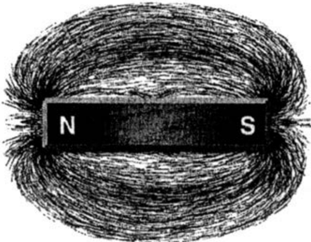
Hình 27. Các đường sức của từ trường. Bột sắt đã vạch nên các đường sức từ nối cực bắc (N) và cực nam (S) của nam châm.
