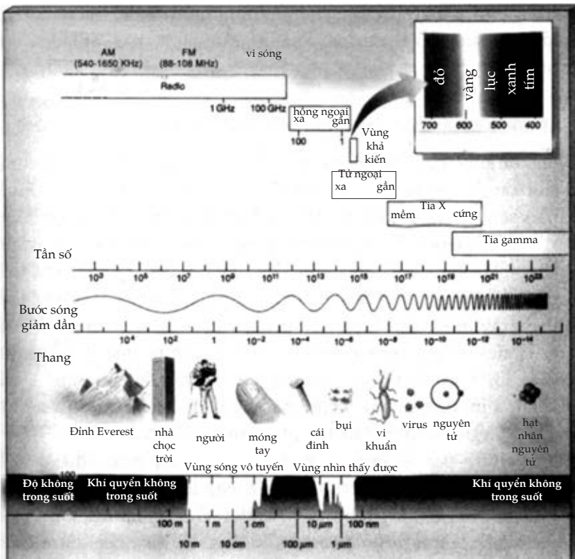
Hình 32. Phổ điện từ . Đó là tập hợp các loại ánh sáng khác nhau. Tính chất duy nhất phân biệt loại ánh sáng này với loại ánh sáng khác chính là bước sóng, tần số hoặc năng lượng của nó. Bước sóng càng dài thì tần số và năng lượng càng nhỏ, và ngược lại. Theo trật tự bước sóng giảm dần (hay tần số và năng lượng tăng dần) ta có: sóng vô tuyến, vi sóng, hồng ngoại, các ánh sáng nhìn thấy được, tia cực tím và các tia X và gamma. Thang tương ứng với bước sóng được minh họa bằng các vật tiêu biểu. Chỉ có các sóng vô tuyến và ánh sáng nhìn thấy được mới có thể xuyên qua dễ dàng khí quyển Trái đất mà không bị hấp thụ (hình dưới). Để thu nhận tất cả các loại ánh sáng, các nhà thiên văn phải đưa lên quỹ đạo các kính thiên văn vượt ra ngoài khí quyển Trái đất.
